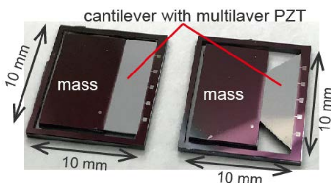
圧電式マイクロ振動発電素子
