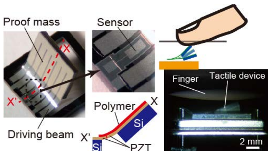
人に振動を与える触覚デバイス・柔軟材料との組合せで実現
